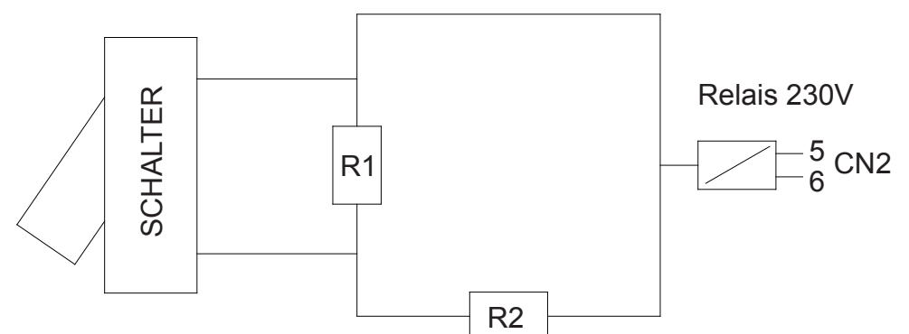
Verdrahtungsplan
